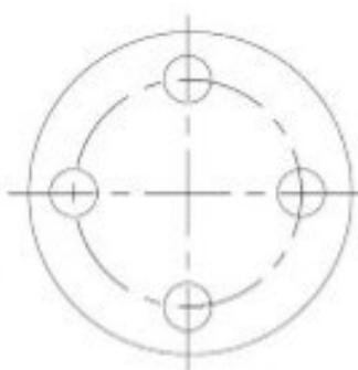
SS316 FLANGE - TABLE E - BLIND
